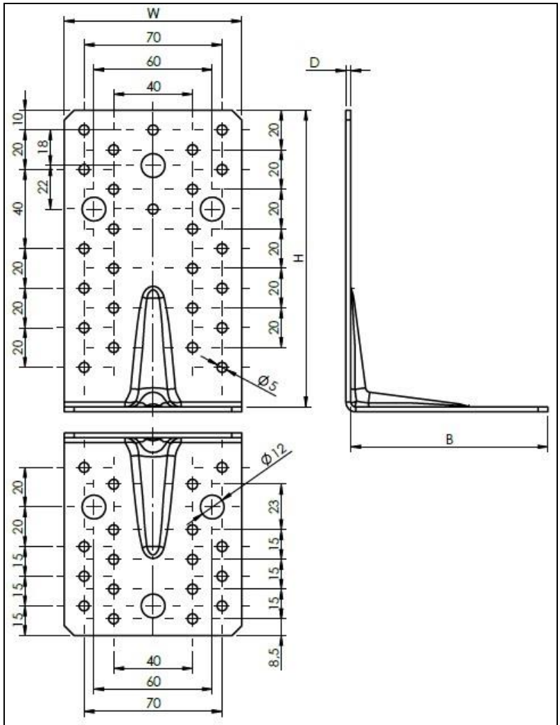
Figure 56 Type KP 10, KPL 10
