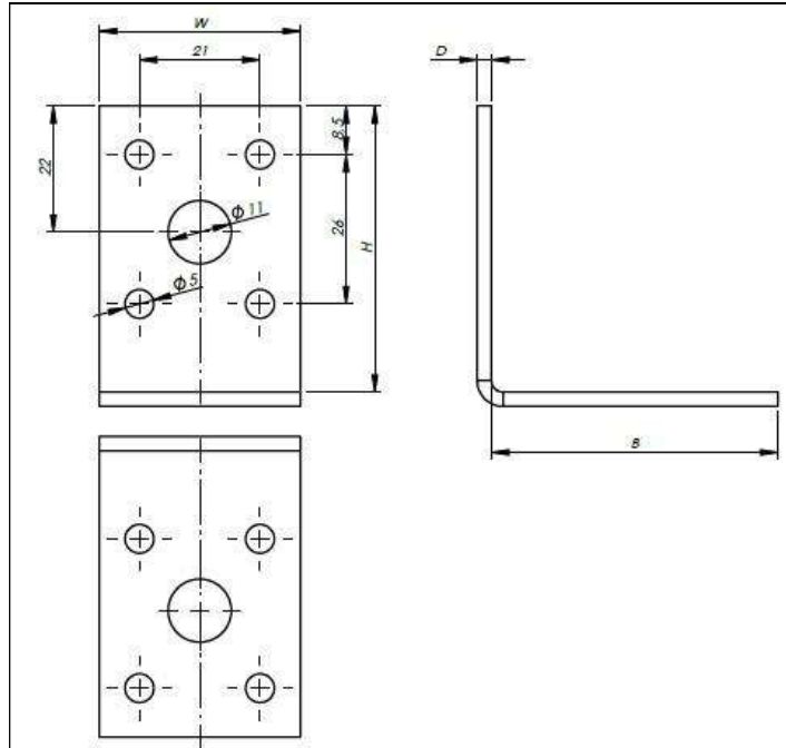
Figure 23 Type KL
