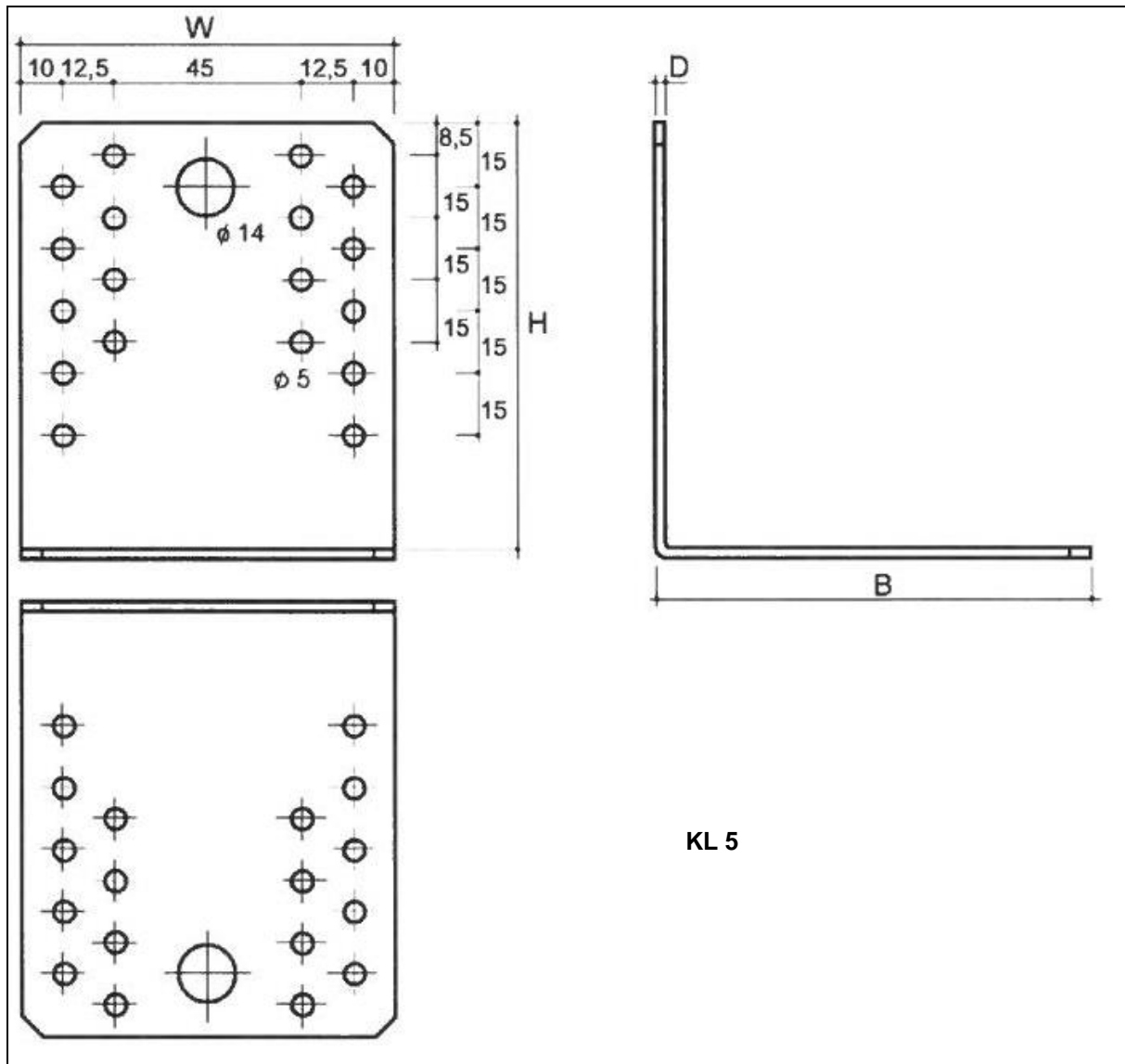
Figure 22 Type KL
